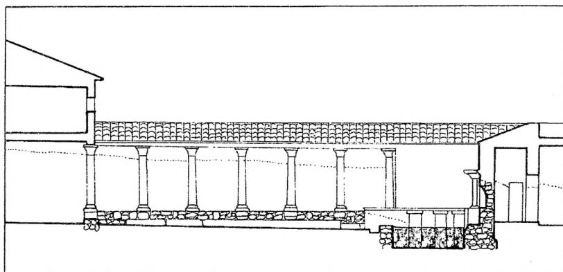
Сл. 3 – Стоби, Куќата на Парсениј , голем перистил, аксонометрија и пресек
