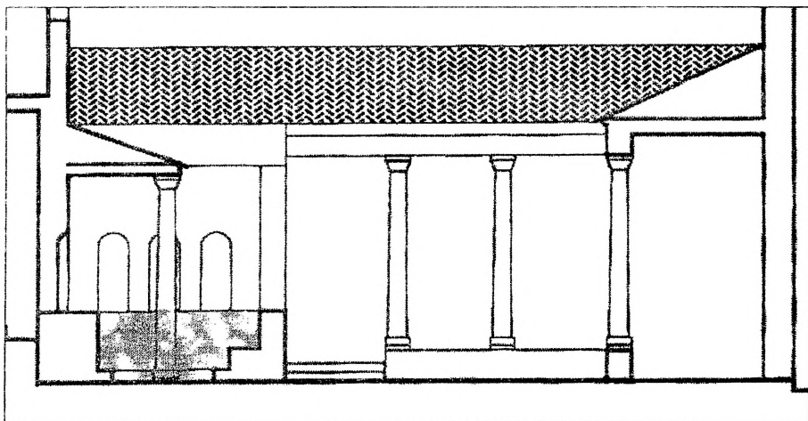
Сл. 7 – Стоби, Куќата на Полихарм, перистил, аксонометрија и пресек
